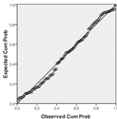
Gambar 1 Uji Normalitas
