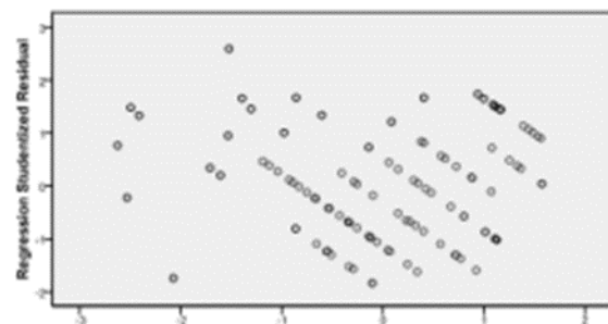
Gambar 3 Uji Heteroskedastisitas
