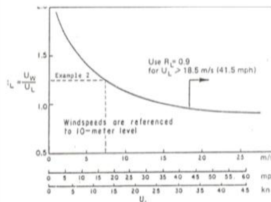
Gambar 2. Hubungan antara kecepatan angin di laut dan darat (Sumber: Bambang Triatmodjo, 1999)
