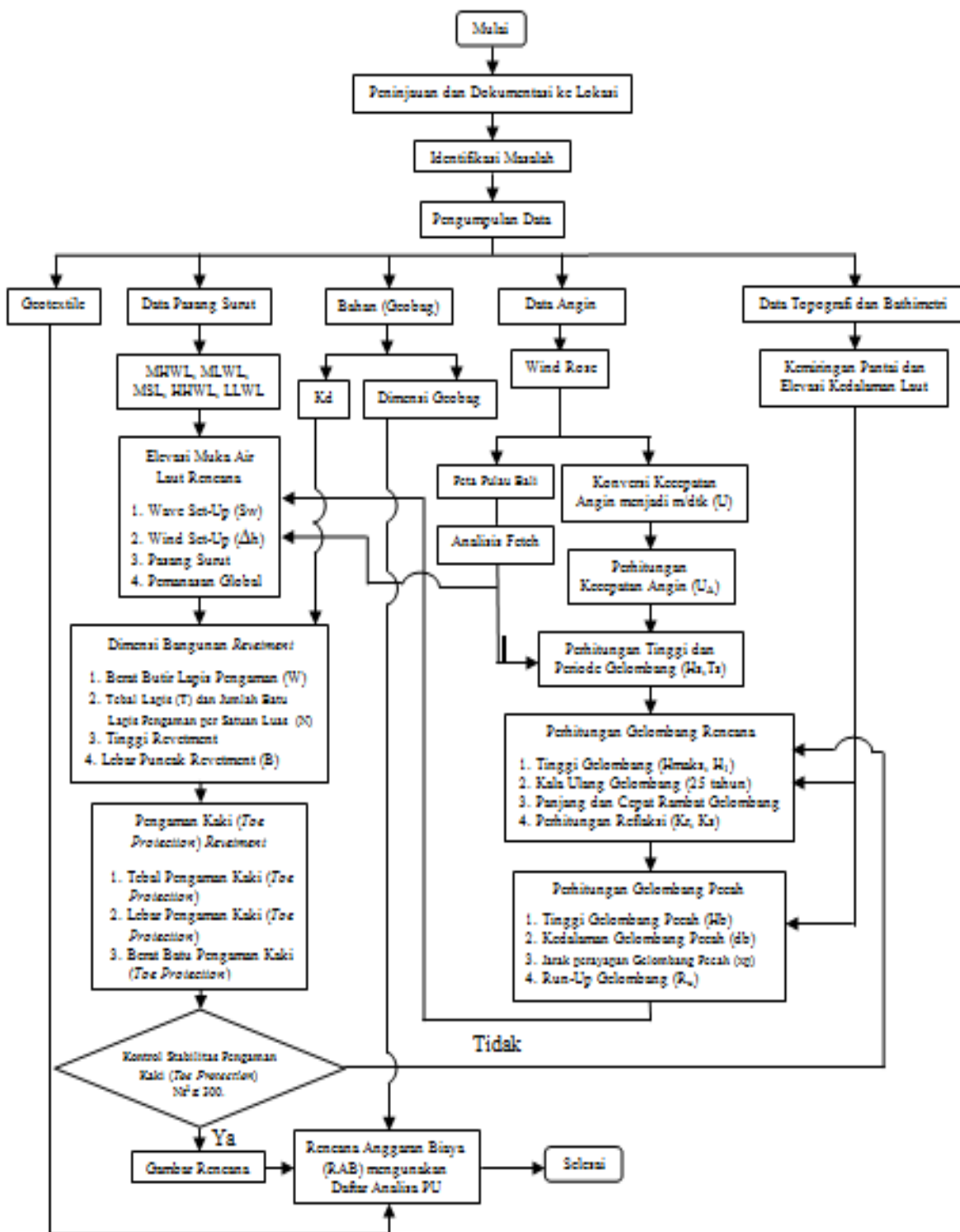
Gambar 4. Skema Perencanaan
